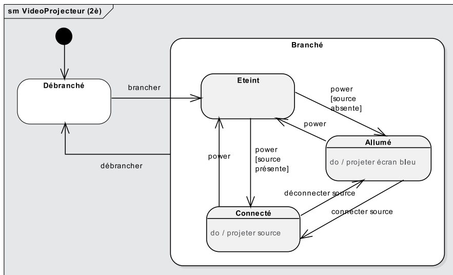
Figure 6-14. Deuxième version du diagramme d'états du vidéoprojecteur
