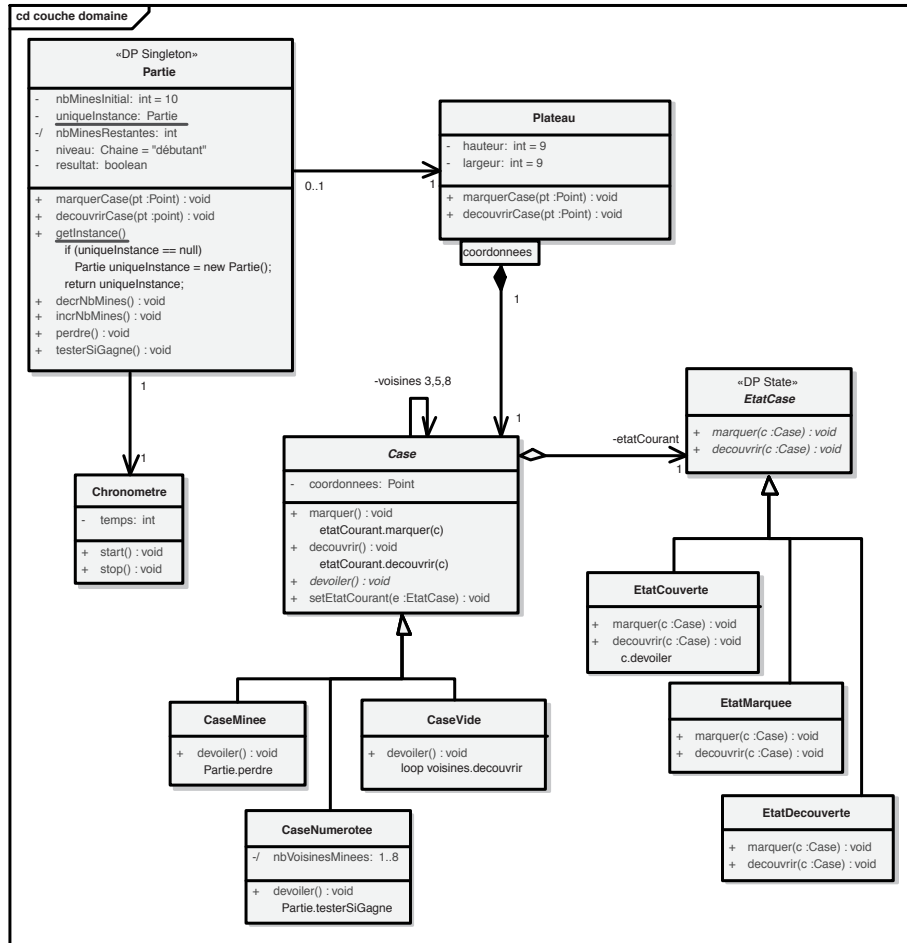
Figure 8-40. Diagramme de classes de conception du jeu de démineur
