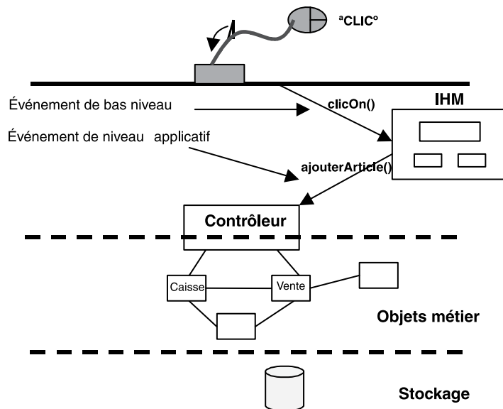
Figure 7-34. Diagramme illustrant l'ajout de l'objet contrôleur
