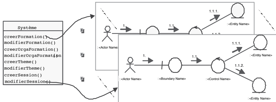
Figure 7-51. Démarche de conception initialisée par les opérations système
