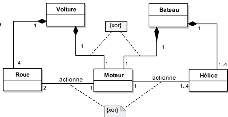
Figure 4-31. Exemple douteux d'associations au même niveau de décomposition
