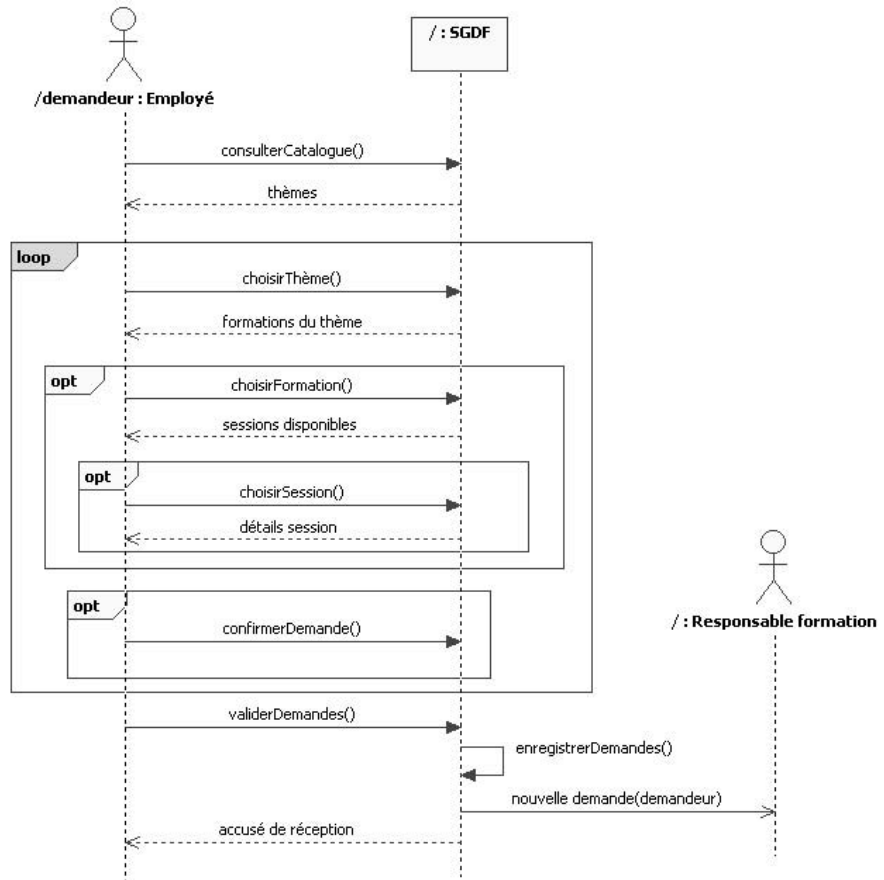
Figure 7-63. Diagramme de séquence système de Demander une formation
