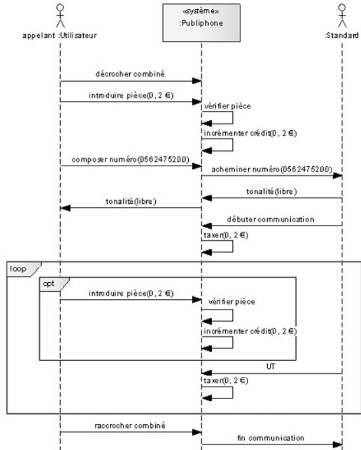
Figure 5-8. Diagramme de séquence système enrichi du scénario nominal de Téléphoner
