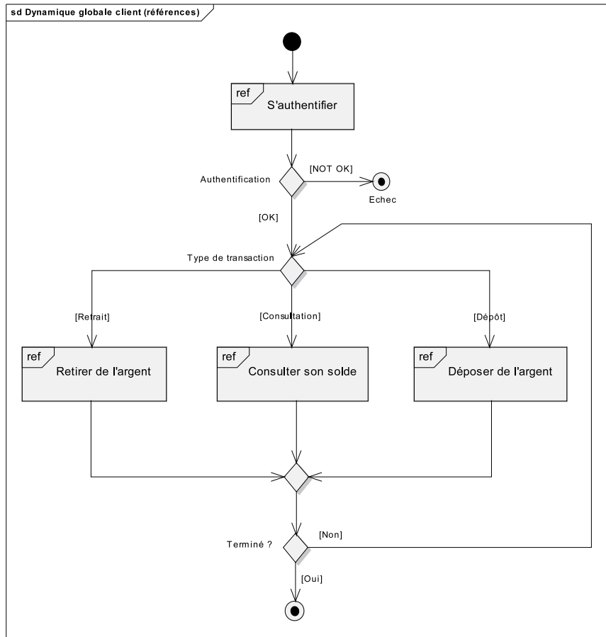
Figure 1-25. Vue d'ensemble des interactions du client banque
