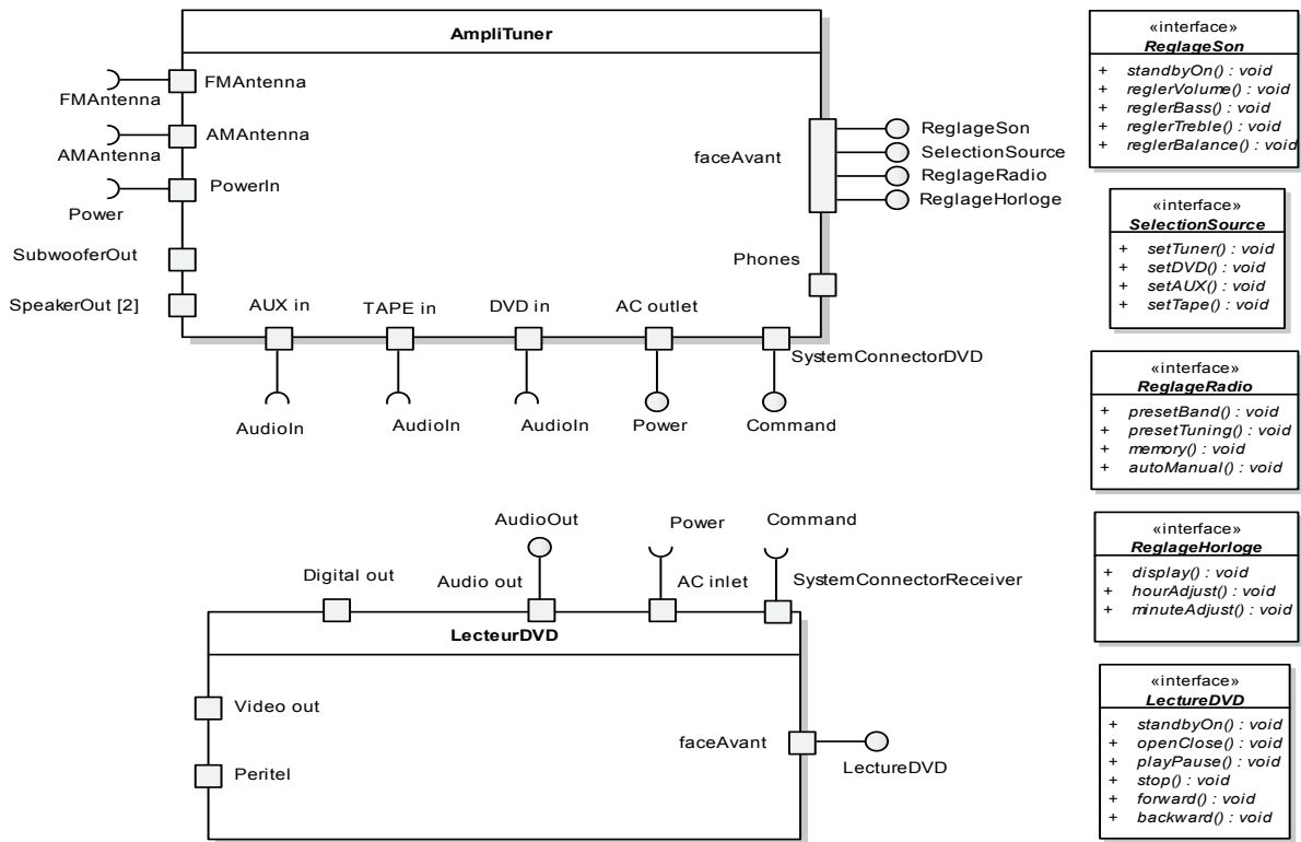
Figure 4-34. Eléments de la chaîne HI-FI
