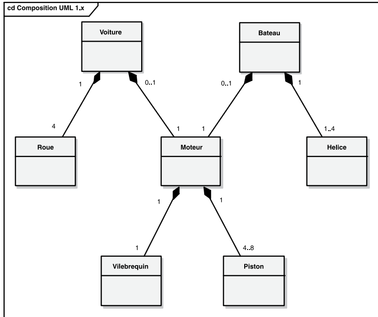
Figure 4-30. Utilisation de la composition UML 1.x
