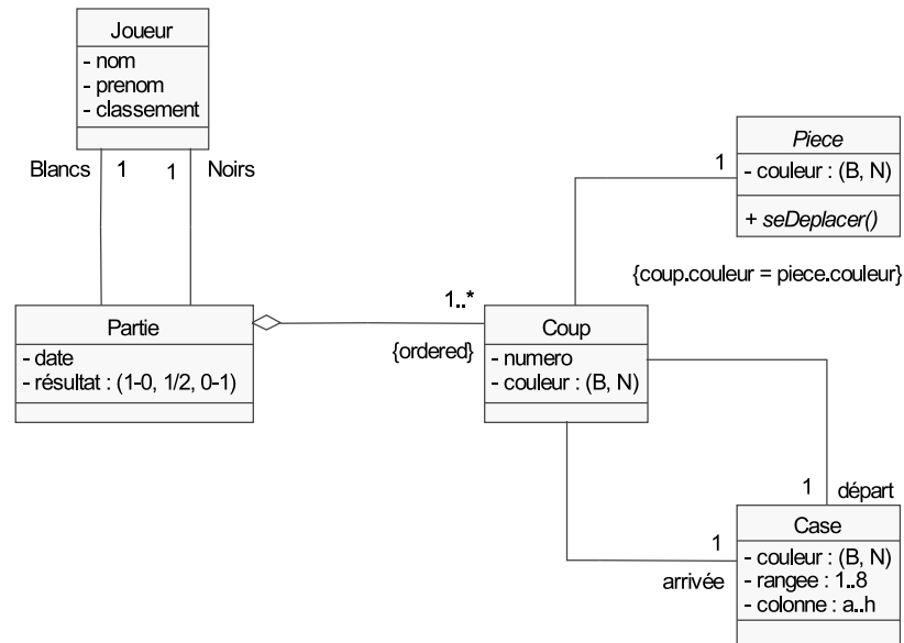
Figure 4-29. Modélisation détaillée du déroulement de la partie
