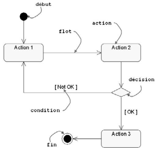
Figure 1-11. Bases du diagramme d'activité UML 2
